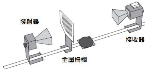
圖九 實驗架設圖II
