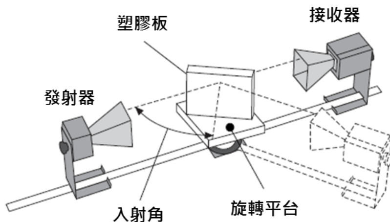
圖十 實驗架設圖 III
