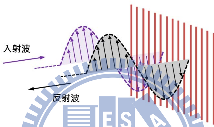
圖三 微波入射金屬柵欄示意圖 (振動方向與金屬柵欄平行)
