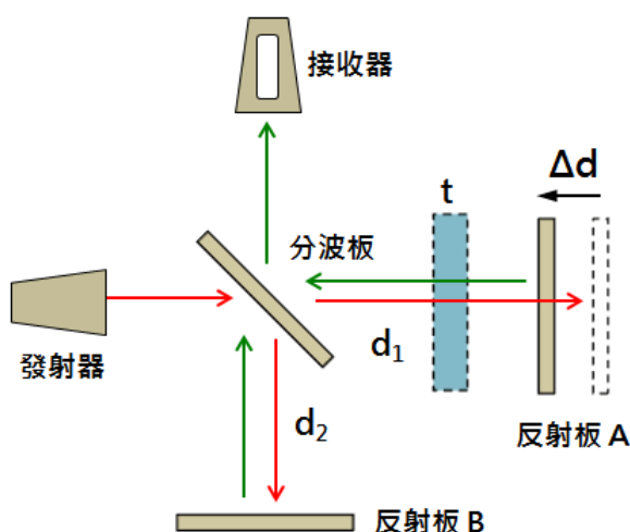
圖六 麥克森干涉示意圖 III
