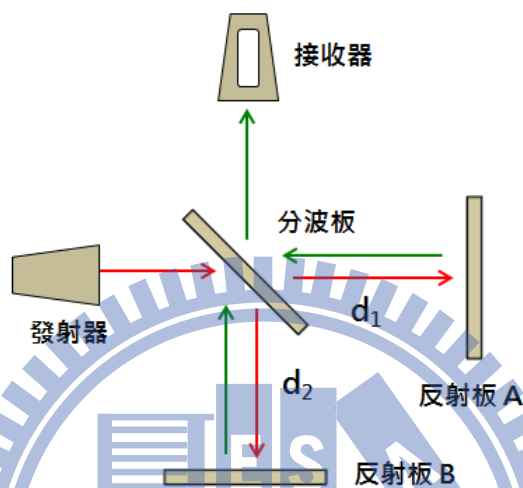
圖四 麥克森干涉示意圖 I
