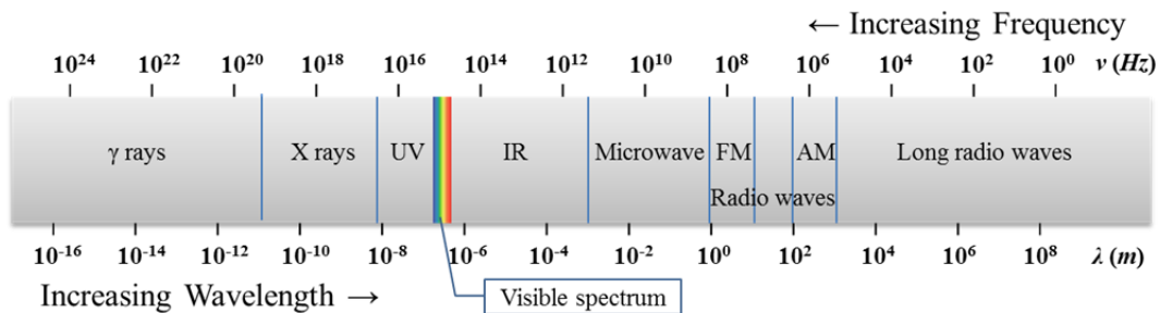
圖二 電磁波頻譜圖
