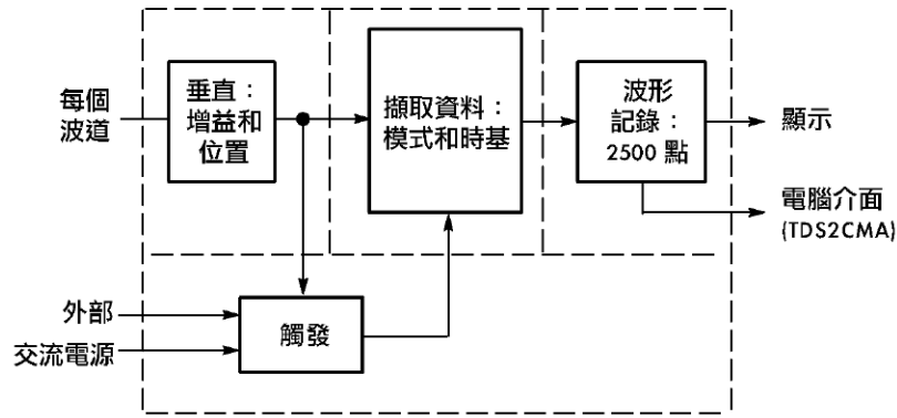
圖一 數位示波器原理
